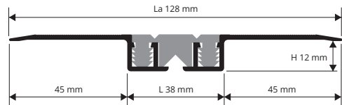
PENF 130... масштаб 1:2
