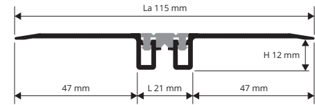
PENF 130... масштаб 1:2
