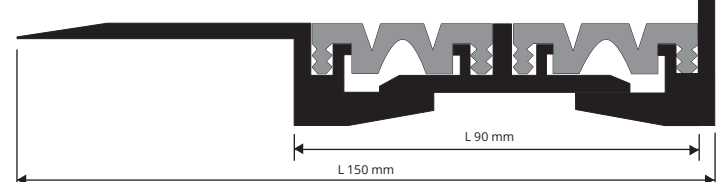
PENFP 210... масштаб 1:2
