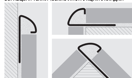
AC - Полированная нерж. сталь AISI 304/1.4301-V2A ACML - Суперблестящий нерж. сталь AISI 304/1.4301-V2A ACS - Сатиновая нерж. сталь AISI 304/1.4301-V2A
