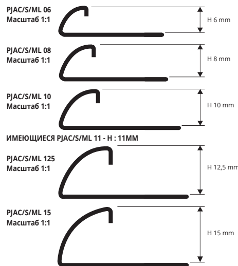
САТИНИРОВАННАЯ НЕРЖ. СТАЛЬ AISI 304/1.4301-V2A с защитной пленкой - длина бруска 2,7 ЛИН.М - упак. 20 шт. - 54 ЛИН.М - 10/10 мм
