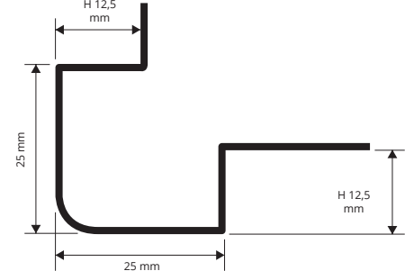
PEBDAC/ACS 125 масштаб 1:1
