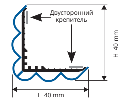
PFC... 40/40A масштаб 1:2
