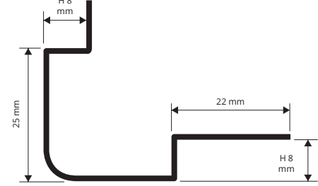
PEBDAC/ACS 10 масштаб 1:1
