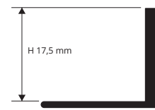
PLGON 175 масштаб 1:1
